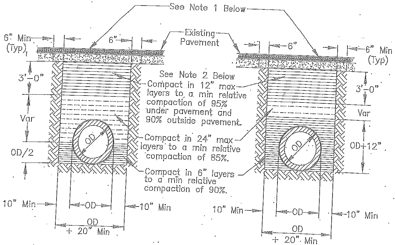
RIGID CONDUIT
